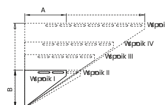
Wsporniki do płyty podstawy i do płyt podpór przejściowych IWSP
