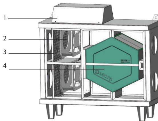
1. obudowa sterownika 2. wentylator 3. filtr G4 4. wymiennik
